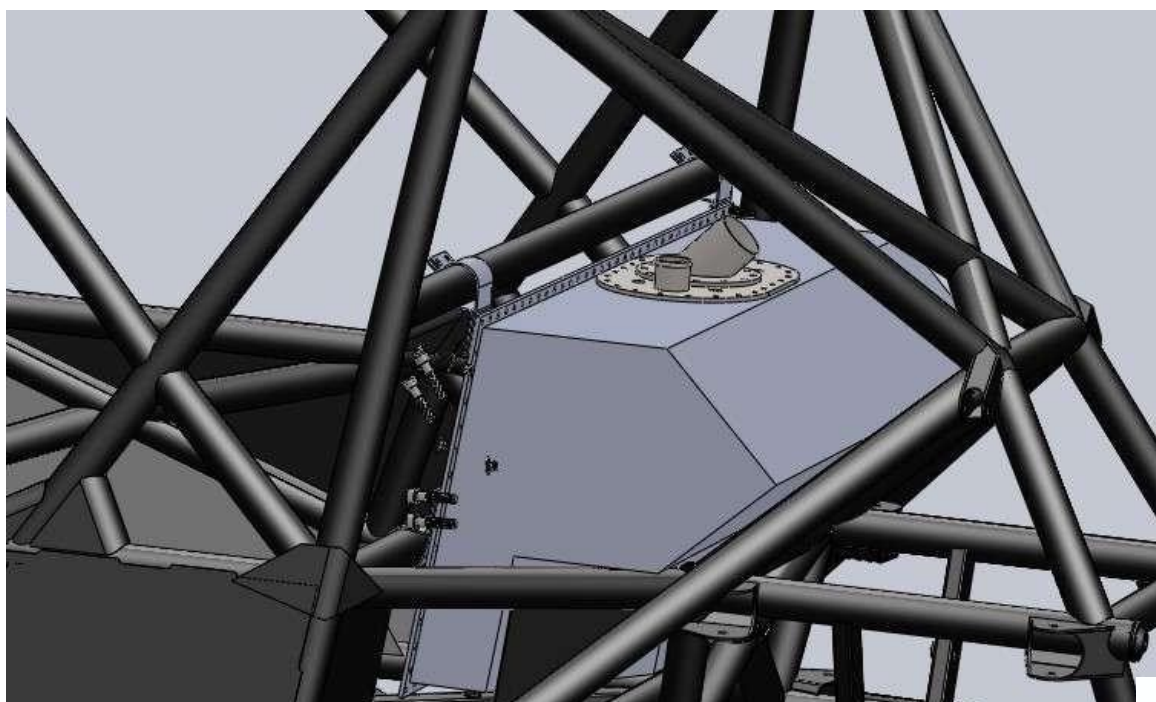
Local do tanque vista isométrica traseira esquerda
