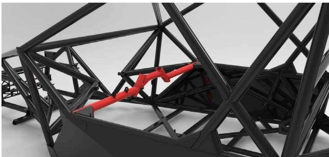
Montagem dos componentes do Chassis
