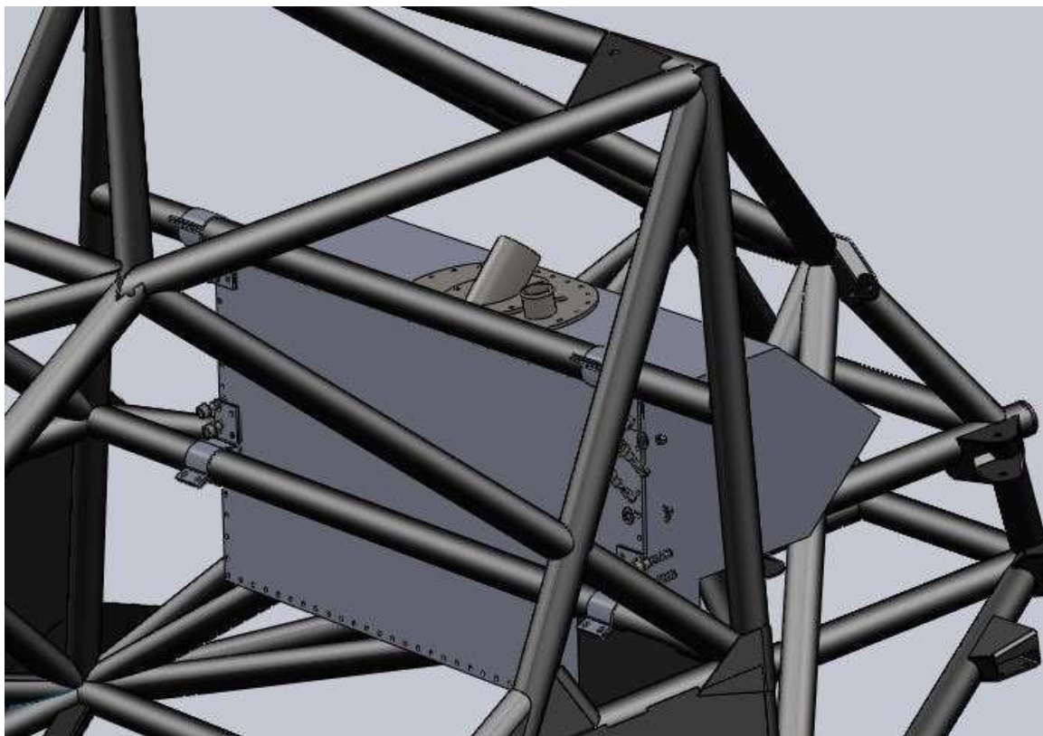
Local do tanque visto de dentro do chassiss
