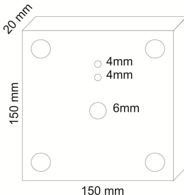
Modelo da placa de acrílico para medição de taxa de compressão
