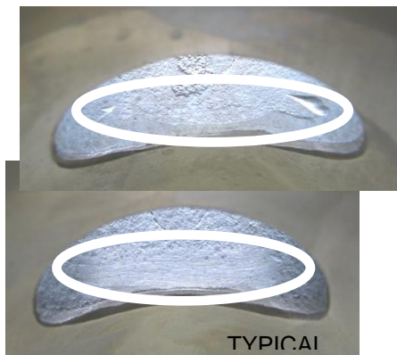
sinais de usinagem (CNC) em combinação com sinais de acabamento
