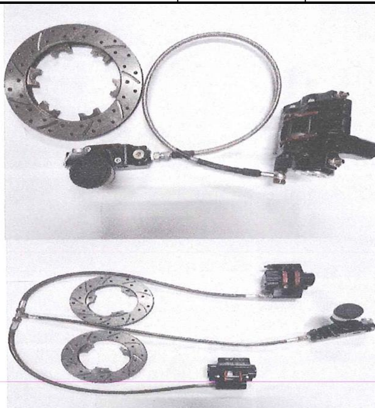
Foto em vista superior do sistema completo
