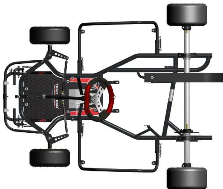
Foto do chassi montado, com pneus
