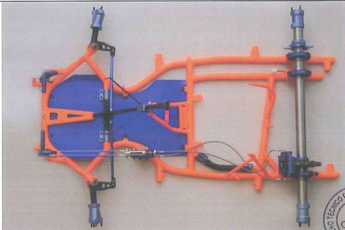
Foto do chassi completo montado, sem carroceria, para-choque, banco e pneus
