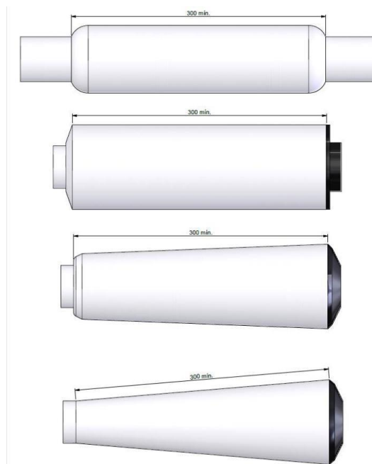
Imagem 5- Método de medição do abafador.
